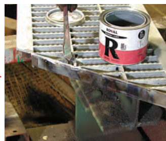
溶接箇所およびフラットバーにローバルを塗装(2回塗りしてください)
